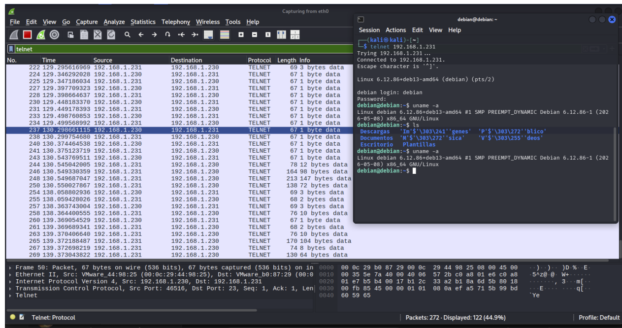
Figura 7: Captura de trafico telnet con Wireshark
