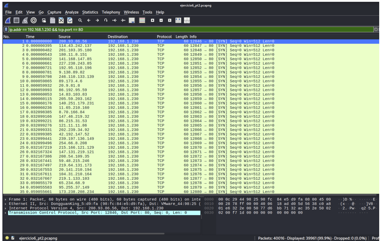
Figura 5: Simulación de ataque DDoS con hping3 y fuentes aleatorias
