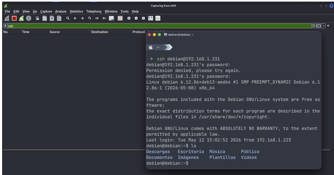
Figura 9: Captura de tráfico ssh con Wireshark
