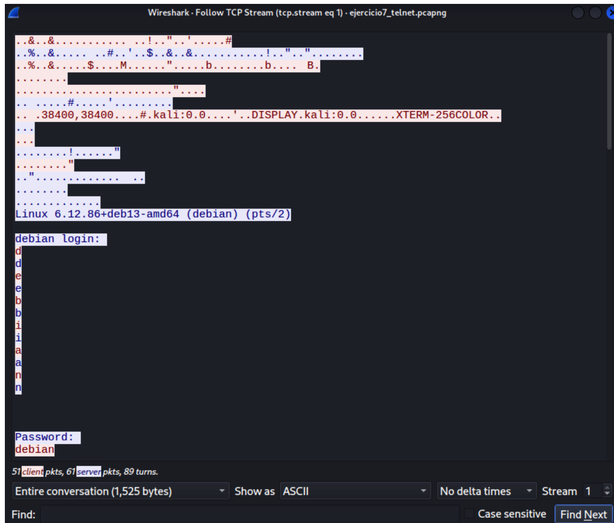
Figura 8: Revisión del payload de un paquete telnet con Wireshark
